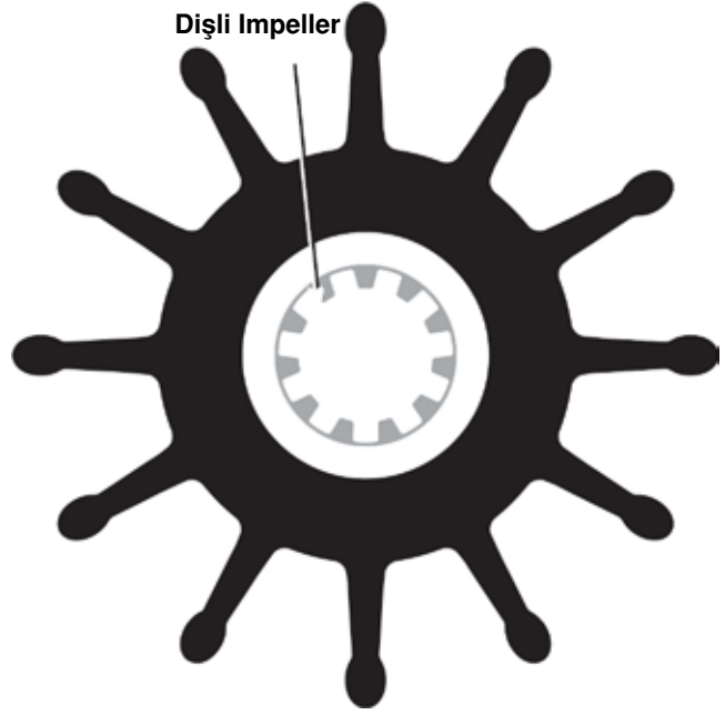
SR11320 Sherwood Impeller 27000K Geniřlik: 73 mm Ø: 84 mm
