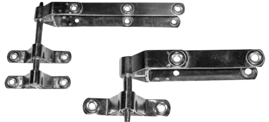
SR20538 Krom İğnecik No:1 Aynakıç Takım SR20540 Krom İğnecik No:1 Bodoslama Takım • 304 Kalite
