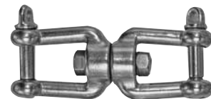
SR22561 Firdöndü Çift Kilitli 5 mm SR22562 Firdöndü Çift Kilitli 6 mm SR22564 Firdöndü Çift Kilitli 8 mm SR22566 Firdöndü Çift Kilitli 10 mm SR22568 Firdöndü Çift Kilitli 12 mm SR22570 Firdöndü Çift Kilitli 16 mm SR22572 Firdöndü Çift Kilitli 19 mm • 304 Kalite
