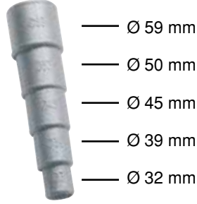
SR10252 Hortum Konnektörü 32-59 mm
