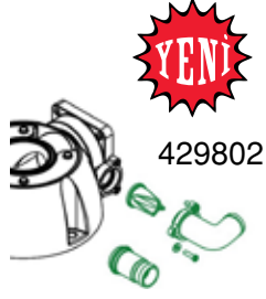
SR08395 TMC Tuvalet Motor Çıkışı 3 Parça
