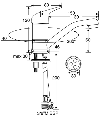
SR08214 Musluk (Sıcak-Soğuk) Barka - MM6700/15 SR08215 Musluk (Sıcak-Soğuk) Barka - MM6700/20
