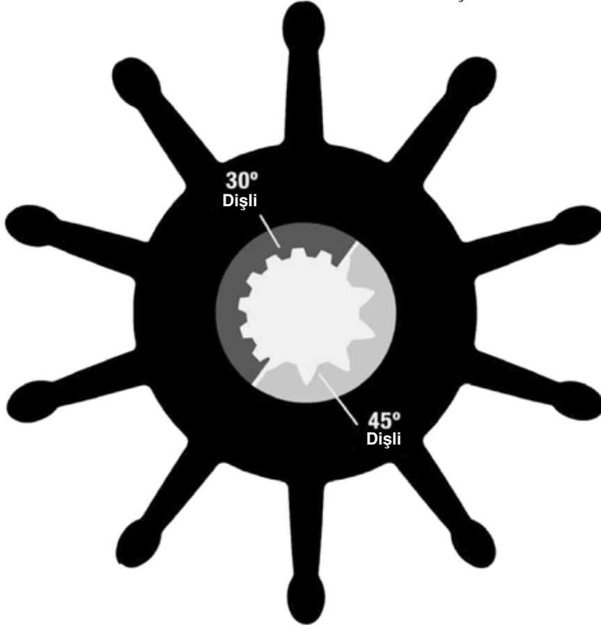
SR11320 Sherwood Impeller 27000K Geniřlik: 73 mm Ø: 84 mm
