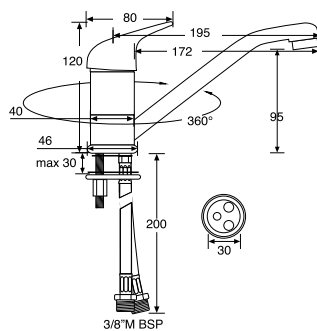
SR08214 Musluk (Sıcak-Soğuk) Barka - MM6700/15 SR08215 Musluk (Sıcak-Soğuk) Barka - MM6700/20
