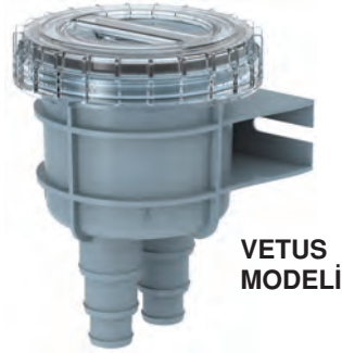
SR10266 Plastik Deniz Suyu Filtresi Vetüs Modeli 13-16-19 mm Ölçüler: Ø:110 mm - Boy: 150 mm SR10268 Plastik Deniz Suyu Filtresi Vetüs Modeli 25-32-38 mm Ölçüler: Ø:150 mm - Boy: 190 mm
