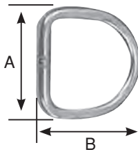
SR23160 Krom D 04 mm - A: 38mm B:33 mm SR23162 Krom D 05 mm - A: 40mm B:35 mm SR23164 Krom D 06 mm - A: 45mm B:35 mm SR23166 Krom D 06 mm - A: 55mm B:40 mm SR23168 Krom D 08 mm - A: 70mm B:60 mm • 304 Kalite
