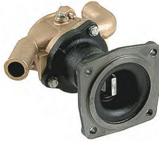
SR11352 Sherwood Deniz Suyu Pompası 1"
