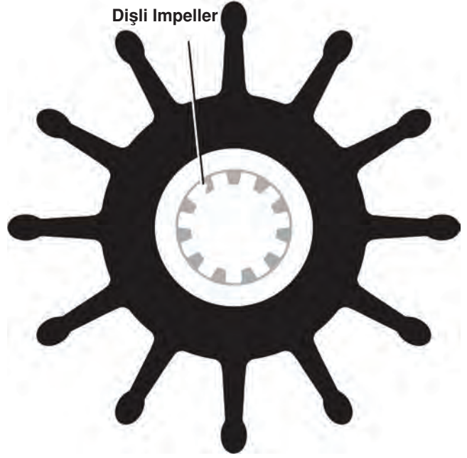
SR11320 Sherwood Impeller 27000K Genişlik: 73 mm Ø: 84 mm
