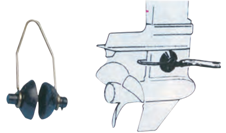
SR02124 Motor Yıkama Aparatı
