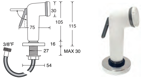
SR08134 Hortumlu Duş (Flanşlı) DS0313
