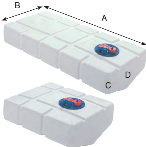
SR18304 Su/Yakıt Tankı - 57 Lt. A: 60, B:50, C:15, D:23 cm SR18306 Su/Yakıt Tankı - 86 Lt. A:107, B:50, C:15, D:23 cm
