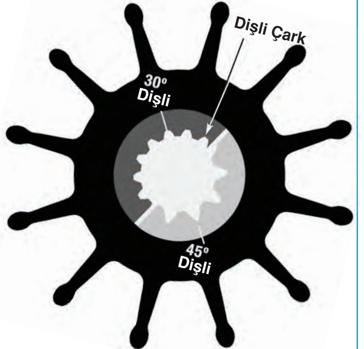
SR11308 Sherwood Impeller 08000K Genişlik: 19 mm Ø: 40 mm
