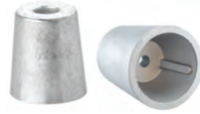
SR29450 Pervane Tutyaş Konik 25 mm SR29452 Pervane Tutyaş Konik 30 mm SR29454 Pervane Tutyaş Konik 35 mm SR29456 Pervane Tutyaş Konik 40 mm SR29458 Pervane Tutyaş Konik 45 mm SR29460 Pervane Tutyaş Konik 50 mm SR29462 Pervane Tutyaş Konik 55 mm SR29464 Pervane Tutyaş Konik 60 mm
