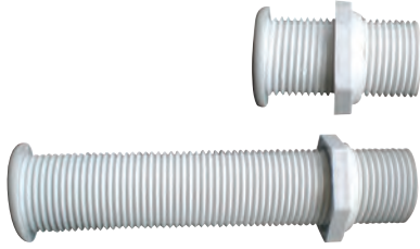
SR18232 Tam Geçişli Dişli Bağlantı Boy: 62 mm SR18233 Tam Geçişli Rekorlu Bağlantı Boy: 100 mm SR18234 Tam Geçişli Dişli Bağlantı Boy: 155 mm Delik Çapları: 25 mm. Beyaz Renk
