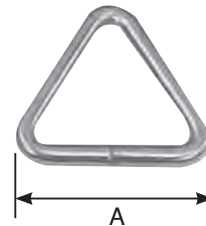
SR23170 Krom Üçgen 04 mm - A: 40x40 mm SR23172 Krom Üçgen 05 mm - A: 50x50 mm SR23174 Krom Üçgen 06 mm - A: 60x60 mm SR23176 Krom Üçgen 08 mm - A: 76x76 mm SR23178 Krom Üçgen 10 mm - A: 99x99 mm • 304 Kalite
