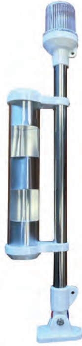
SR14165 Işıklı Bayrak Direği 50 cm Radar Reflektörlü 12 V - Led
