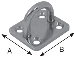
SR21715 Mapa 4 Delikli 5 mm - A: 30mm B:35 mm SR21716 Mapa 4 Delikli 6 mm - A: 33mm B:40 mm SR21718 Mapa 4 Delikli 8 mm - A: 38mm B:50 mm • 304 Kalite
