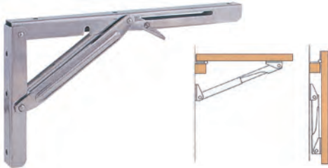
SR19216 Masa ve Oturak Braketi 150 Kg SR19218 Masa ve Oturak Braketi 250 Kg En: 170 mm Boy: 300 mm • 304 Kalite
