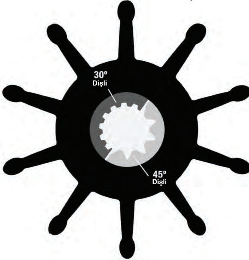
SR11320 Sherwood Impeller 27000K Genişlik: 73 mm Ø: 84 mm
