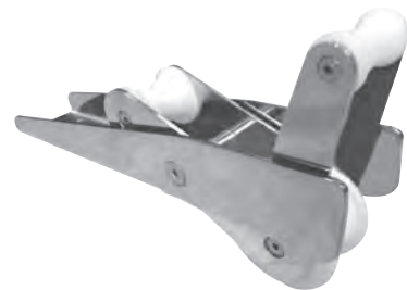
SR20232 Mafsalı Burun Makarası 75 x 400 mm SR20233 Mafsalı Burun Makarası 75 x 500 mm SR20234 Mafsalı Burun Makarası 75 x 600 mm SR20235 Mafsalı Burun Makarası 110 x 600 mm SR20236 Mafsalı Burun Makarası 110 x 700 mm Not: Delta Çapalara Uygundur • 316 Kalite
