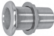
SR27740 Bağlantı Kovanı 3/8" CR-NI SR27742 Bağlantı Kovanı 1/2" CR-NI SR27744 Bağlantı Kovanı 3/4" CR-NI SR27746 Bağlantı Kovanı 1" CR-NI SR27748 Bağlantı Kovanı 1.1/4" CR-NI SR27750 Bağlantı Kovanı 1.1/2" CR-NI SR27752 Bağlantı Kovanı 2" CR-NI
