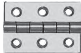
SR23110 Mentese 3,3 x 4 cm • 304 Kalite SR23112 Mentese 4,2 x 6 cm • 304 Kalite SR23114 Mentese 6,0 x 8 cm • 304 Kalite SR23116 Mentese 6,8 x 10 cm • 316 Kalite
