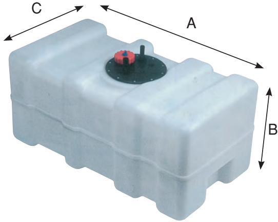
SR18280 Su Tankı - 42 litre A:50, B:30, C:35 SR18282 Su Tankı - 55 litre A:65, B:30, C:35 SR18284 Su Tankı - 70 litre A:80, B:30, C:35
