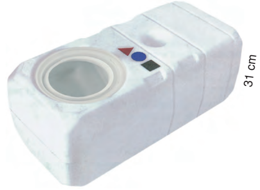
SR18730 Plastik Tank - 49 Lt. Ölçüler: 50x36x31 cm SR18732 Plastik Tank - 64 Lt. Ölçüler: 65x36x31 cm SR18734 Plastik Tank - 78 Lt. Ölçüler: 80x36x31 cm SR18736 Plastik Tank - 93 Lt. Ölçüler: 95x36x31 cm SR18738 Plastik Tank - 108 Lt. Ölçüler: 110x36x31 cm
