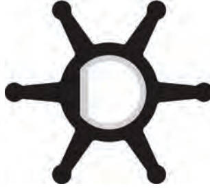
SR11308 Sherwood Impeller 08000K Genişlik: 19 mm Ø: 40 mm
