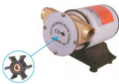
SR09710 Seaflo Güverte Yıkama Pompası 30 Lt. 12 V SR09712 Seaflo Güverte Yıkama Pompası 30 Lt. 24 V • 3 mt. yüksekliğe basar • Tatlı ve deniz suyu ile çalışır. • Ø: 19 mm • Impeller İle Çalışır
